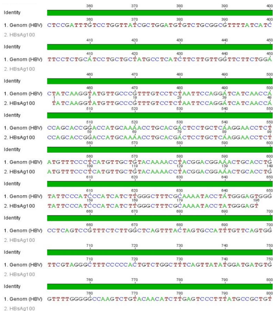
Gambar 4. Alignment sekuen gen insert (penyandi antigen HBsAg100 ) dengan bagian genom virus Hepatitis B (VHB)
