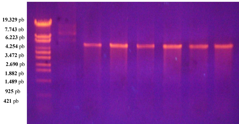
Gambar 3. Pita DNA plasmid pGEX-4T-2 rekombinan hasil elektroforesis dalam 1% agrosa M : marker DNA \lambda . Lajur 1 : Pita DNA plasmid utuh pGEX-4T-2 rekombinan. Lajur 2, 3, 4, 5, 6, 7 : pita DNA plasmid pGEX-4T-2 rekombinan yang dipotong dengan enzim Sma 1.
